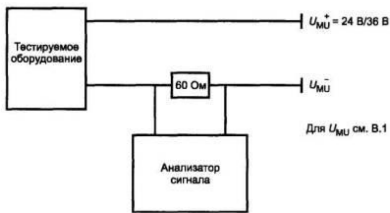
Рисунок А.1 - Оборудование для тестирования качества сигнала при передаче
