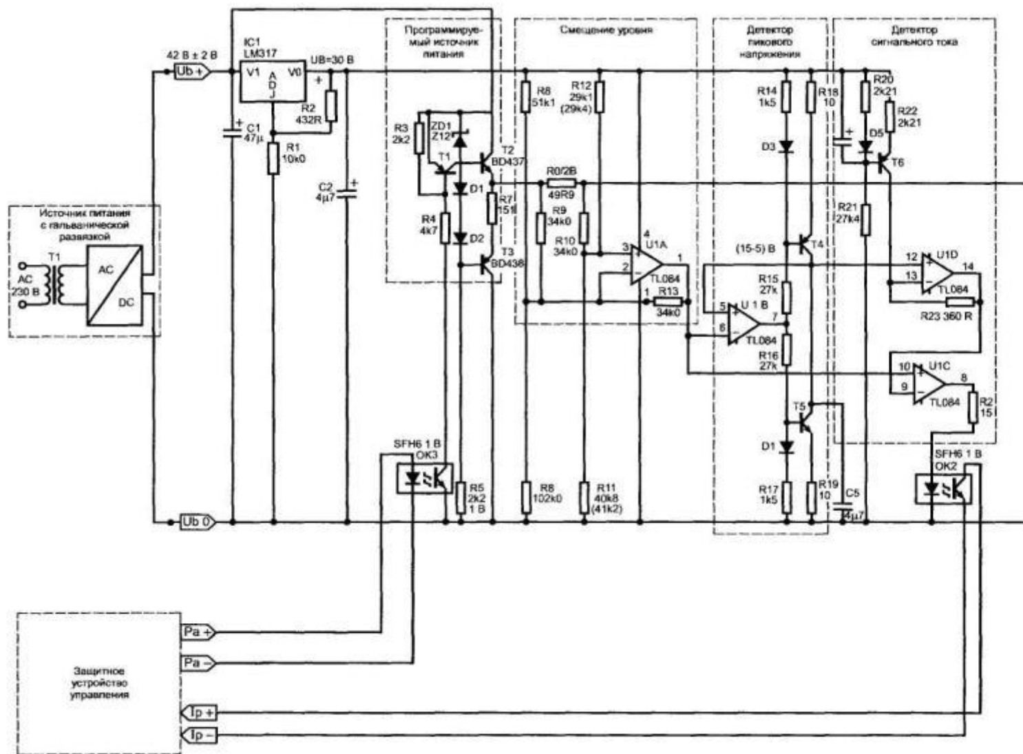
Рисунок С.2 - Конвертер среднего уровня
