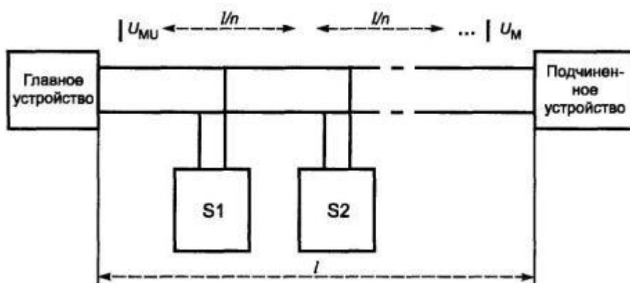
Рисунок В.3 - Тестовое оборудование для М-Bus (I)
