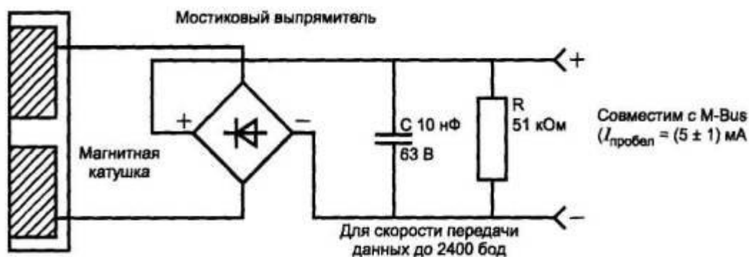
Рисунок 4 - Электрические элементы в теплосчетчике
