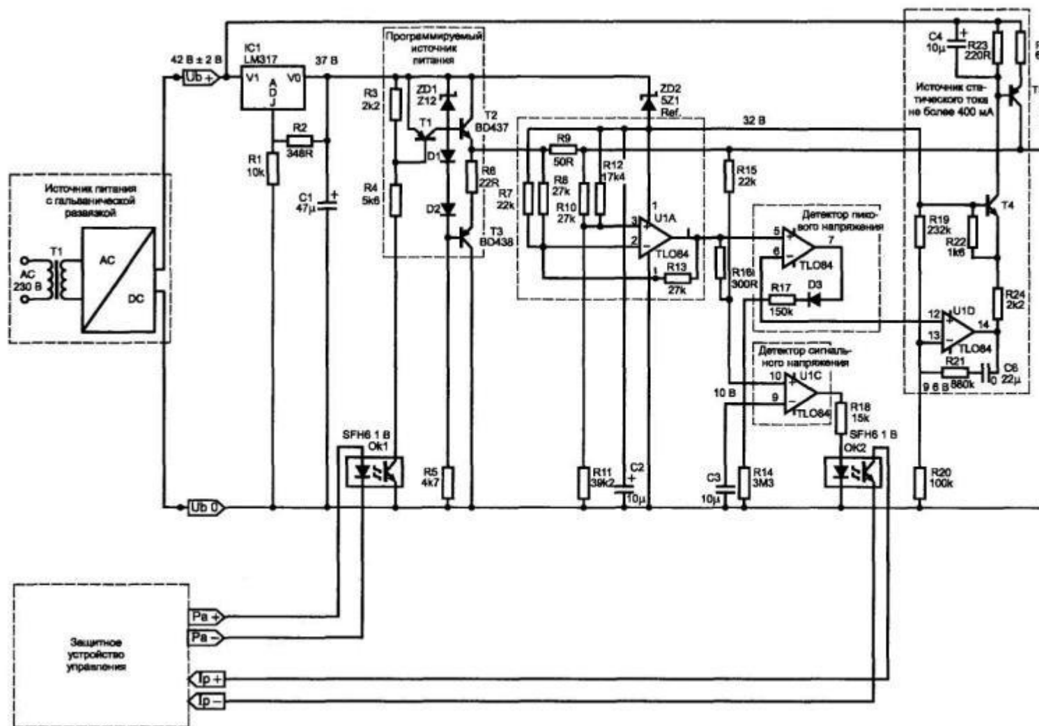
Рисунок С.3 - Конвертер уровней в полном объеме
