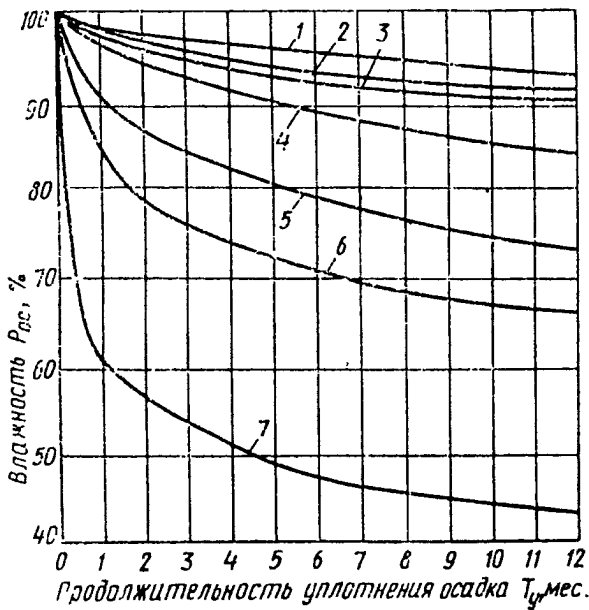
Рис. 3. Средние значения влажности осадка станций осветления и обезжелезивания воды при уплотнении до одного года
