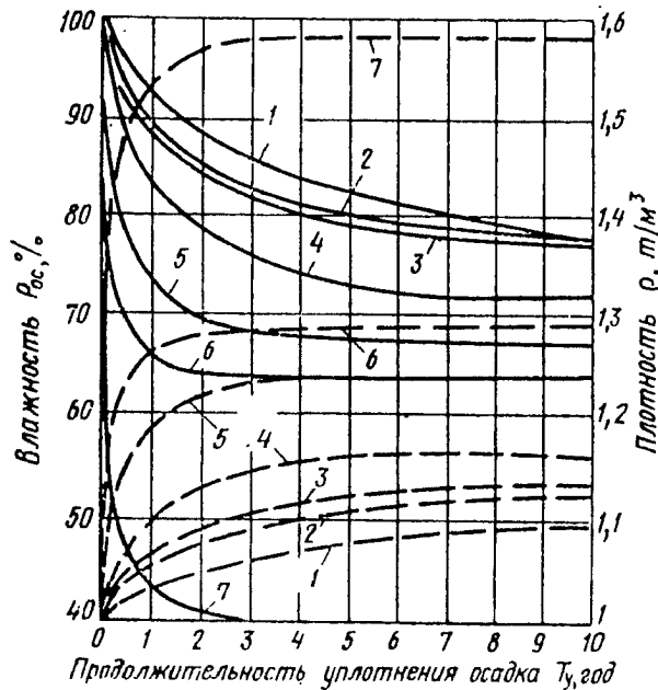
Рис. 1. Средние значения влажности и плотности осадка станций осветления и обеззараживания воды при многолетнем уплотнении
