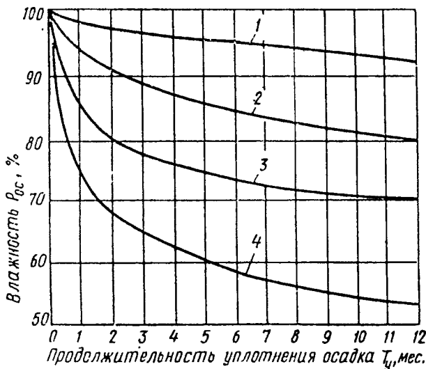
Рис. 4. Средние значения влажности осадка станций обезжелезивания и реагентного умягчения воды при уплотнении до одного года
